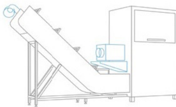
Direkter Ladeausgangskanal in den 1100-L-Behlter mit Staubpartikelfiltrationssystem
